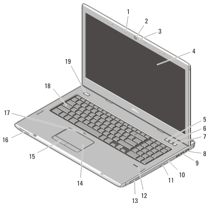
図 7. Vostro 3750 — 正面図
